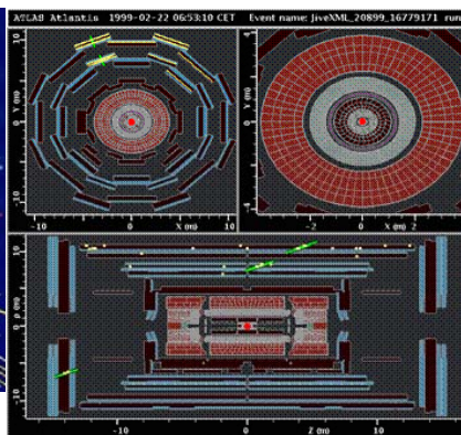
(2) H \rightarrow ZZ^* \rightarrow 4\text{leptons}
