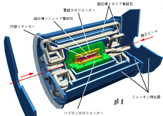
アトラス実験装置
