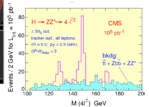
(2) H \rightarrow ZZ^* \rightarrow 4\text{leptons}
