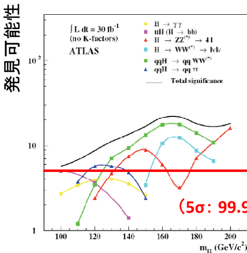
1-4 SM Higgsの発見能力
