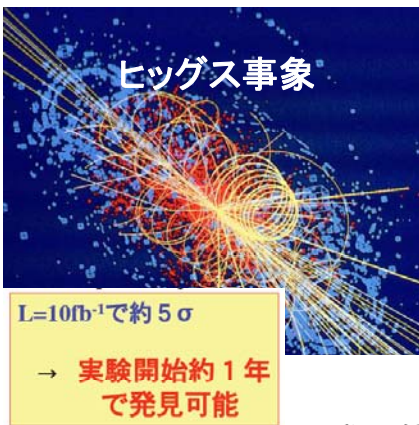
1-4 SM Higgsの発見能力
