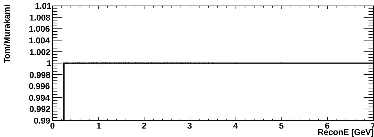
erec_int_nue_ccpi
