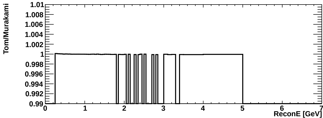
erec_int_signue_ccpi
