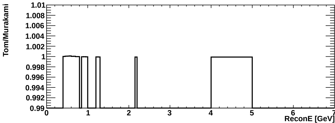
erec_int_signue_cccoh
