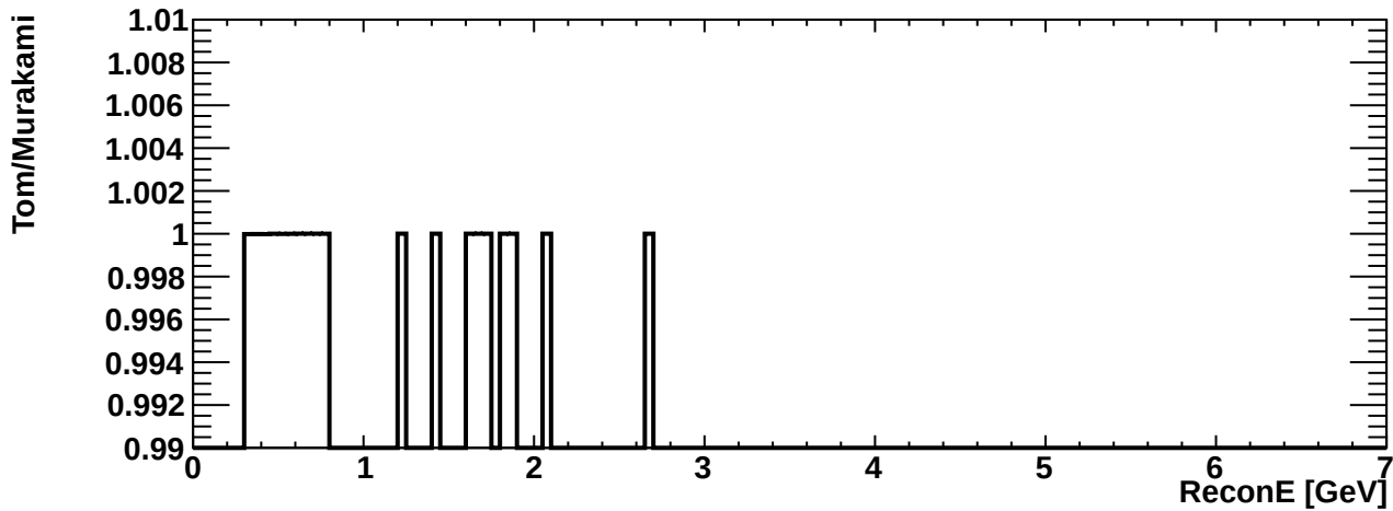
erec_int_nue_cccoh
