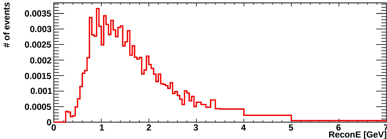
erec_int_numb_cccoh
