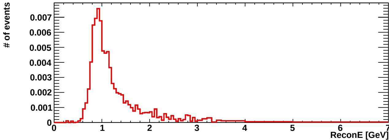
erec_int_signue_ccqe
