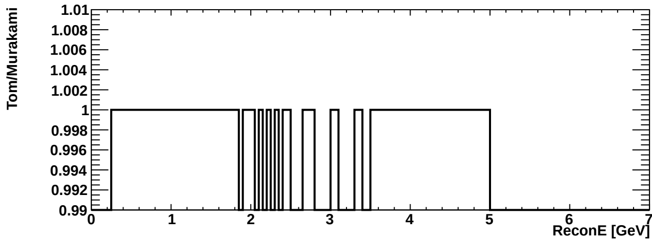
erec_int_nue_ncoth
