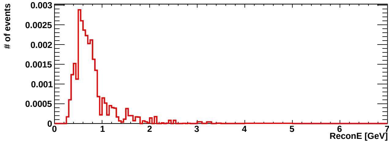
erec_int_signue_ccpi
