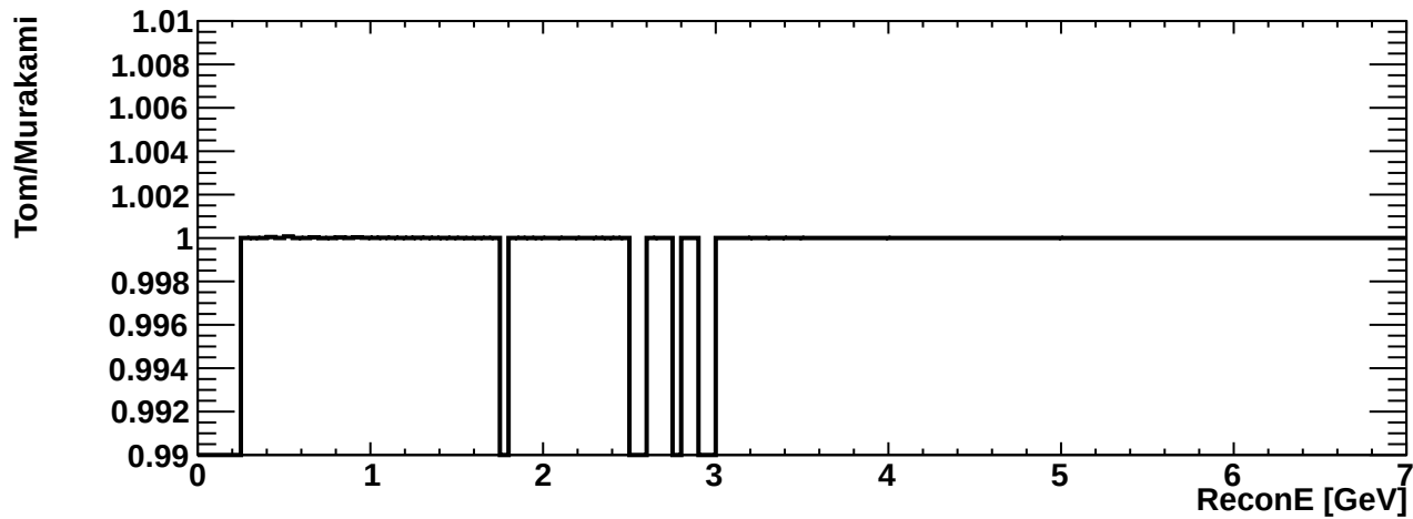
erec_int_nueb_ccpi
