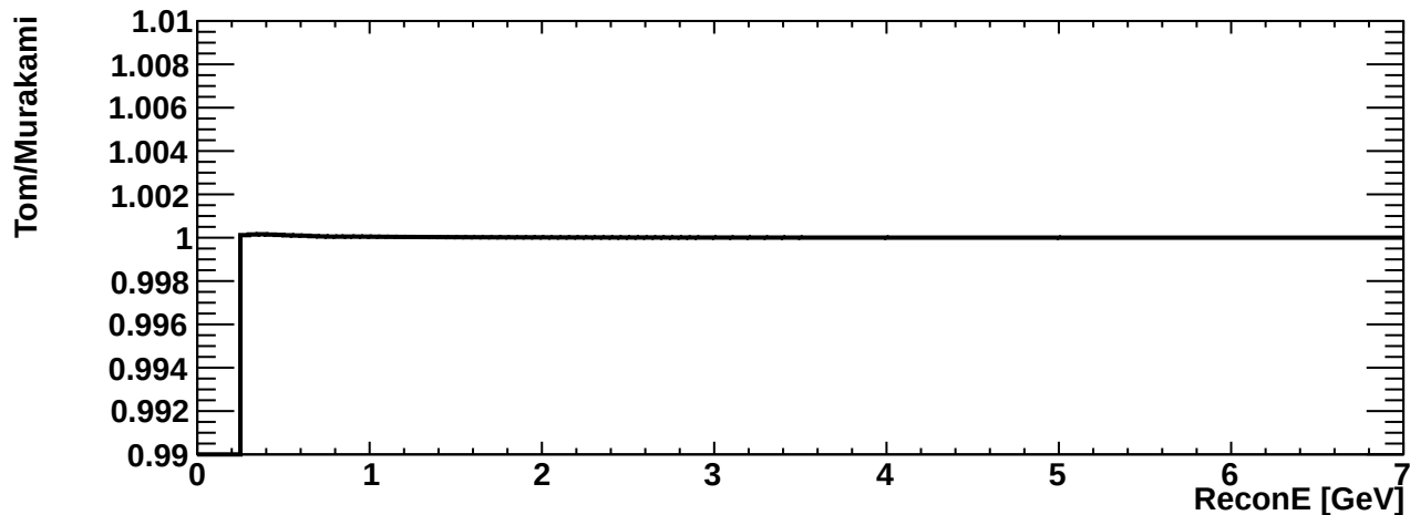
erec_int_numb_ccpi
