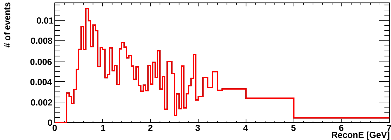
erec_int_numu_cccoh
