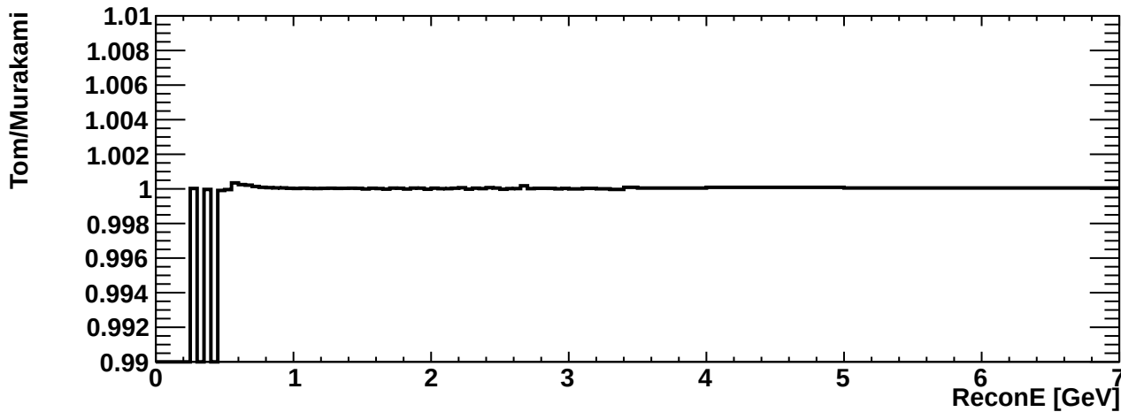
erec_int_signue_ccqe
