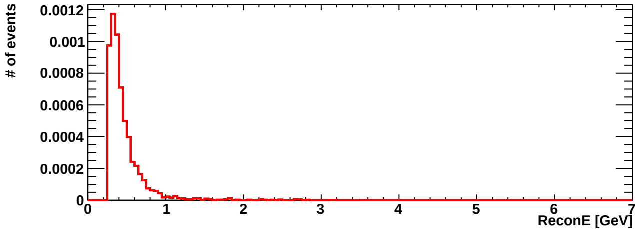
erec_int_nueb_ncoth
