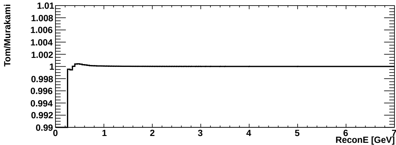
erec_int_numu_cccoh
