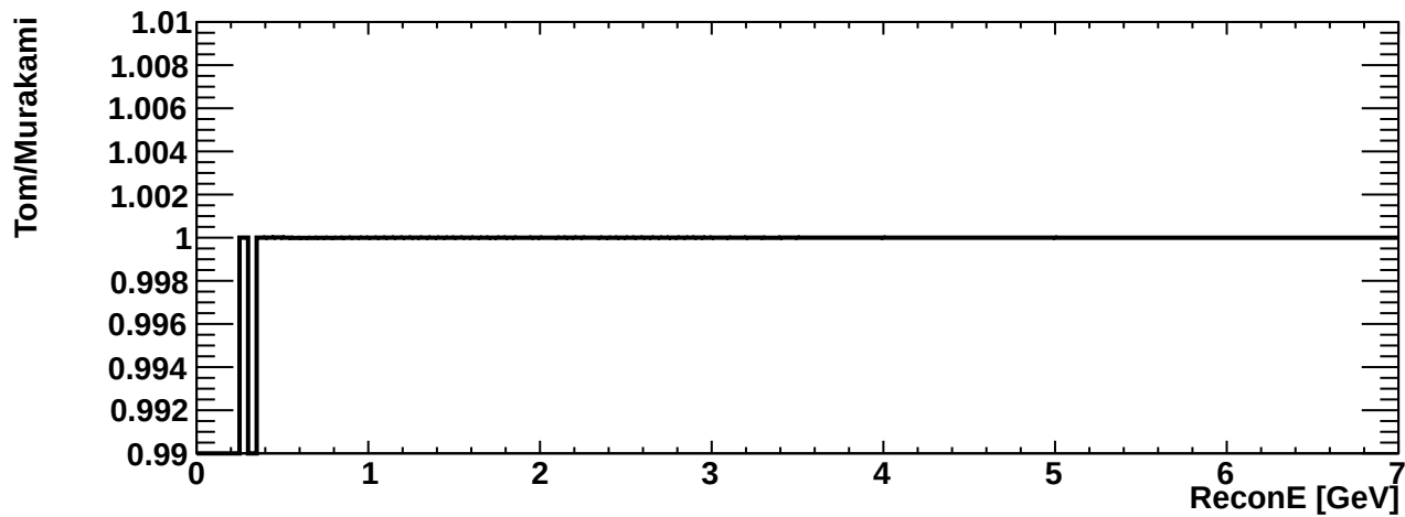
erec_int_nue_ccqe
