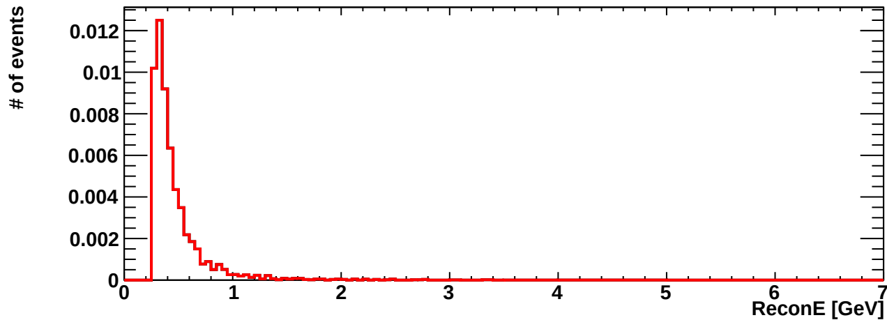
erec_int_nue_ncoth
