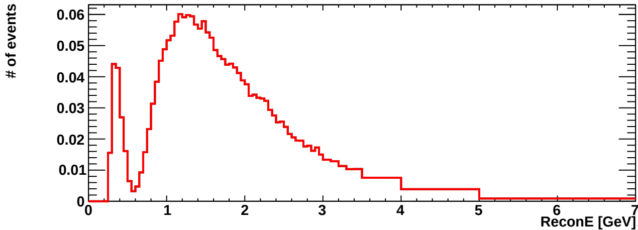
erec_int_numb_ccqe
