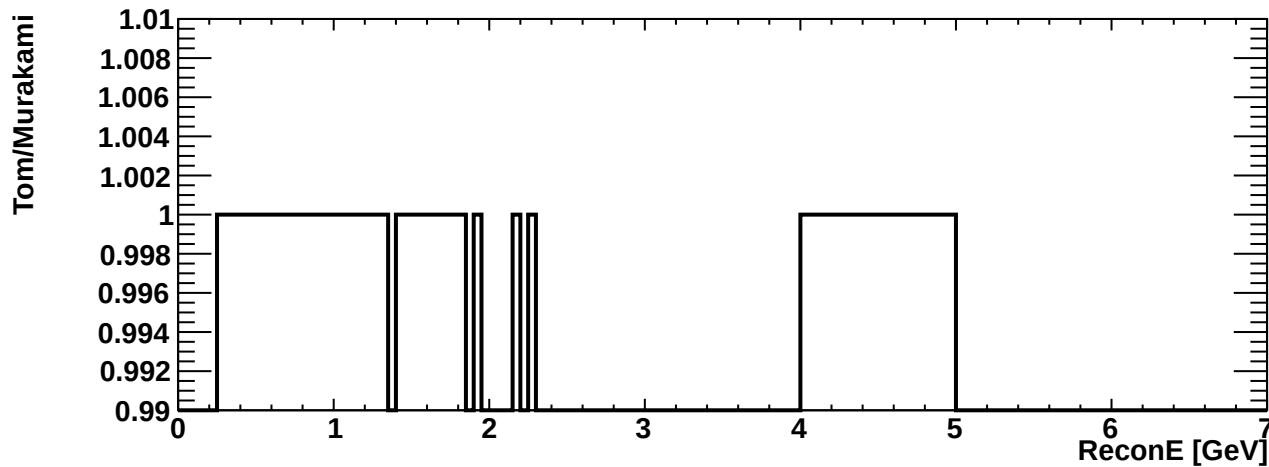
erec_int_nueb_ncpi
