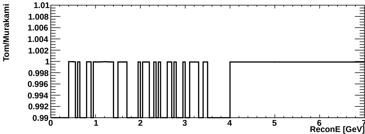
erec_int_signue_ccloth
