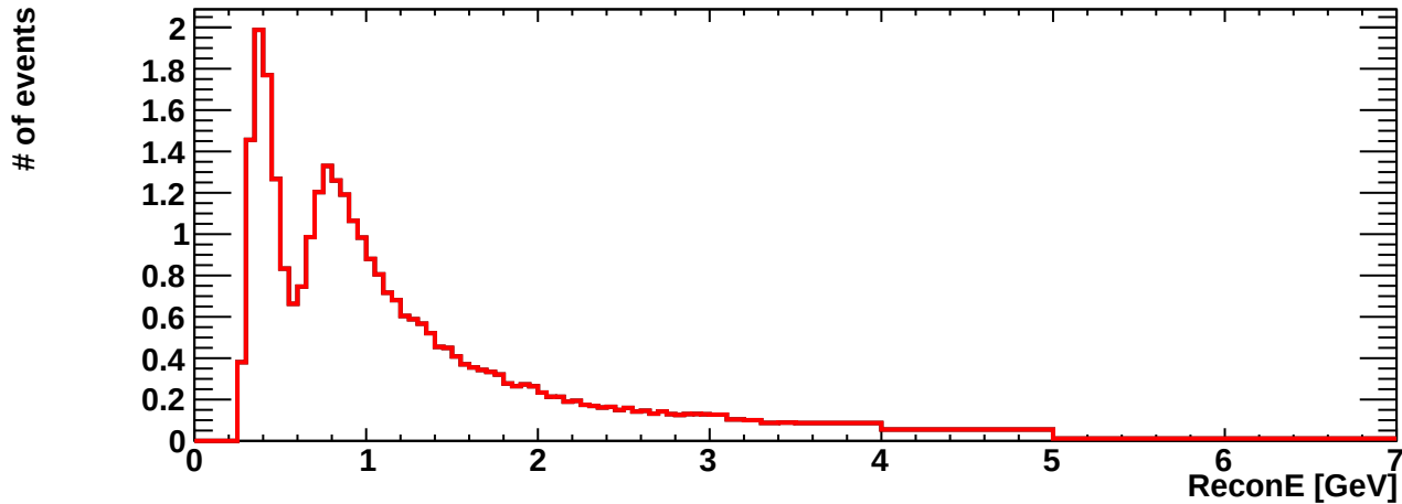
erec_int_numu_ccqe
