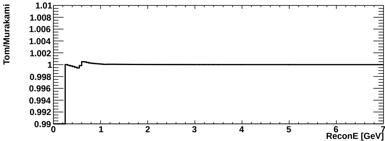
erec_int_numb_ccqe
