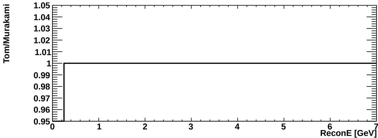
erec_int_numb_cccoh
