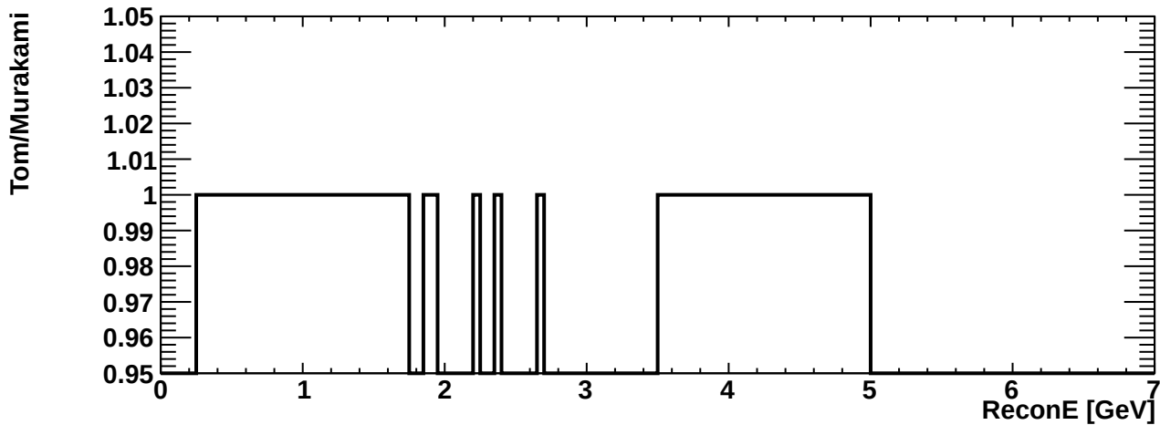
erec_int_numb_ncoth
