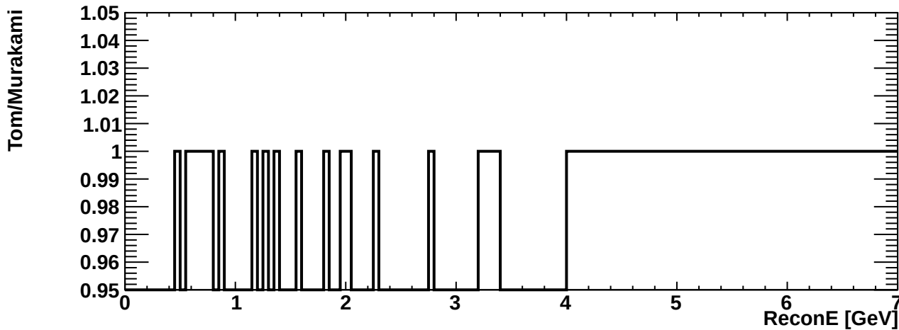
erec_int_nueb_cccoh
