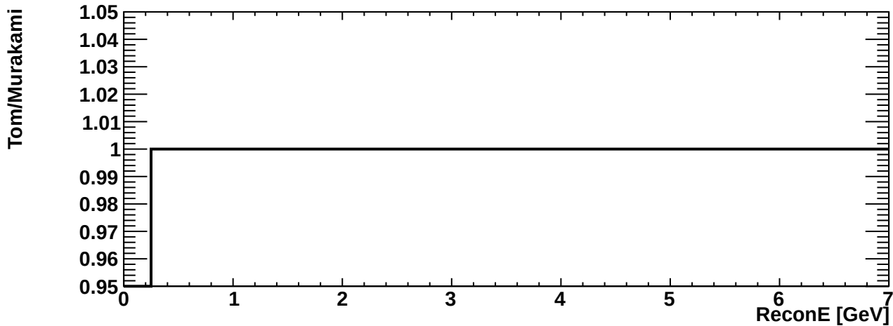
erec_int_numb_ccqe
