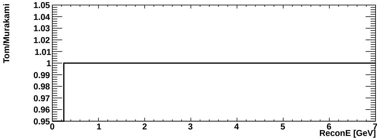
erec_int_numu_cccoh
