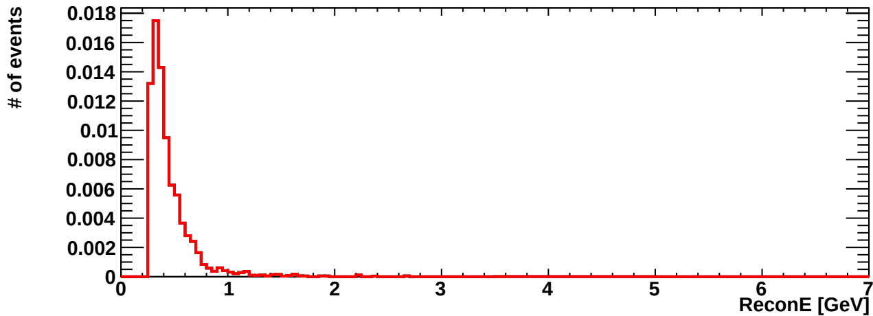
erec_int_numb_ncoth
