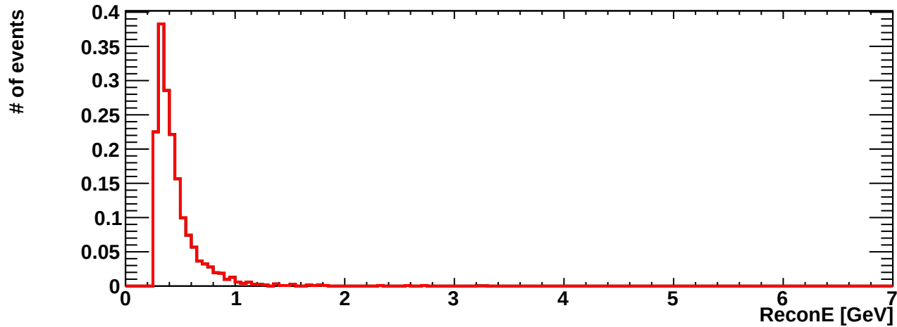
erec_int_numu_ncpi
