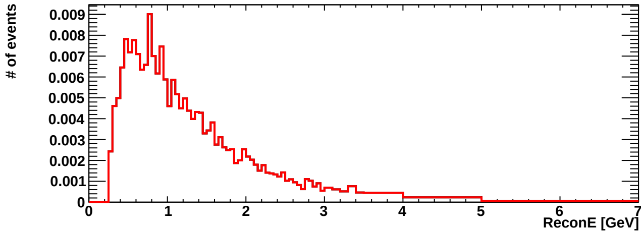
erec_int_numb_cccoh
