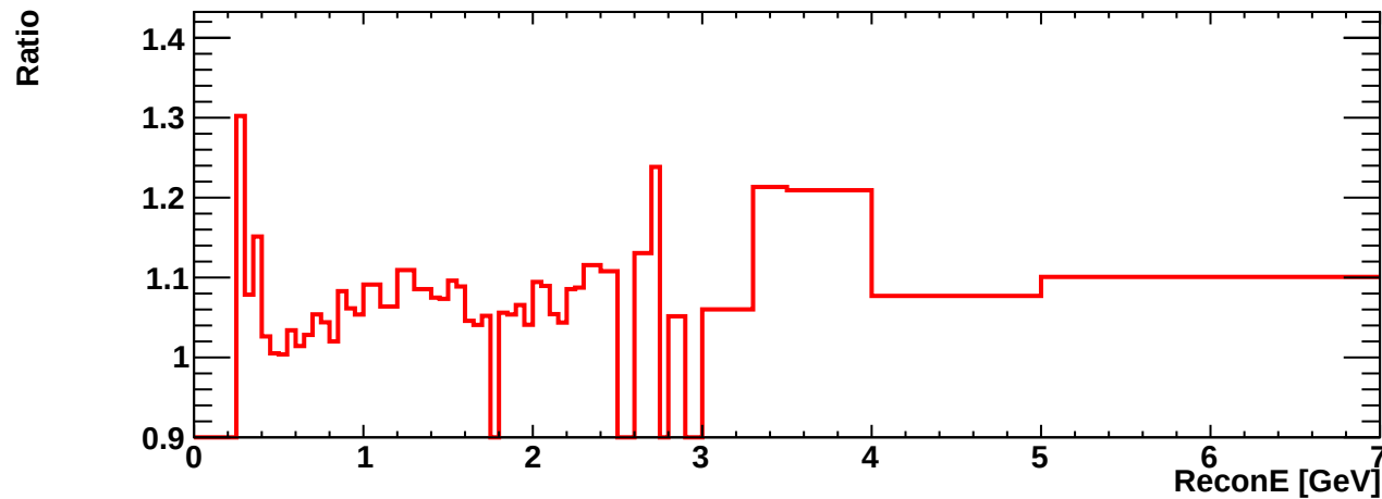
SK nueb ccpi Recon. Energy Spectrum
