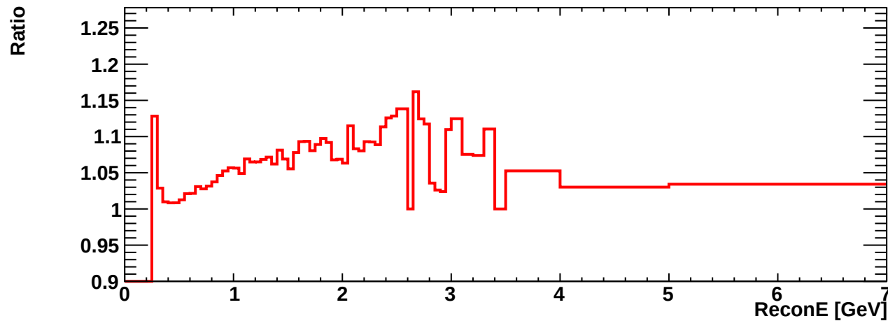
SK nue ccpi Recon. Energy Spectrum
