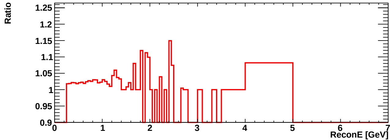
SK nue ncoth Recon. Energy Spectrum
