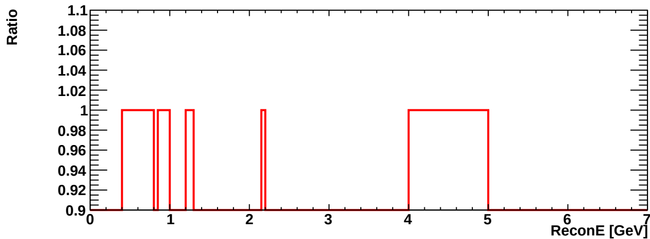
SK signue ccoch Recon. Energy Spectrum
