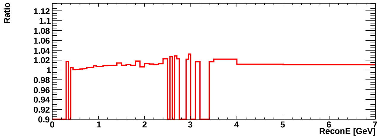
SK nueb ccqe Recon. Energy Spectrum
