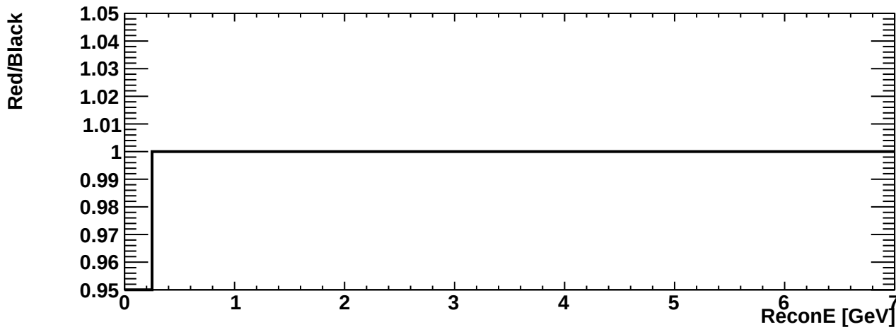
erec_int_numb_cccoh
