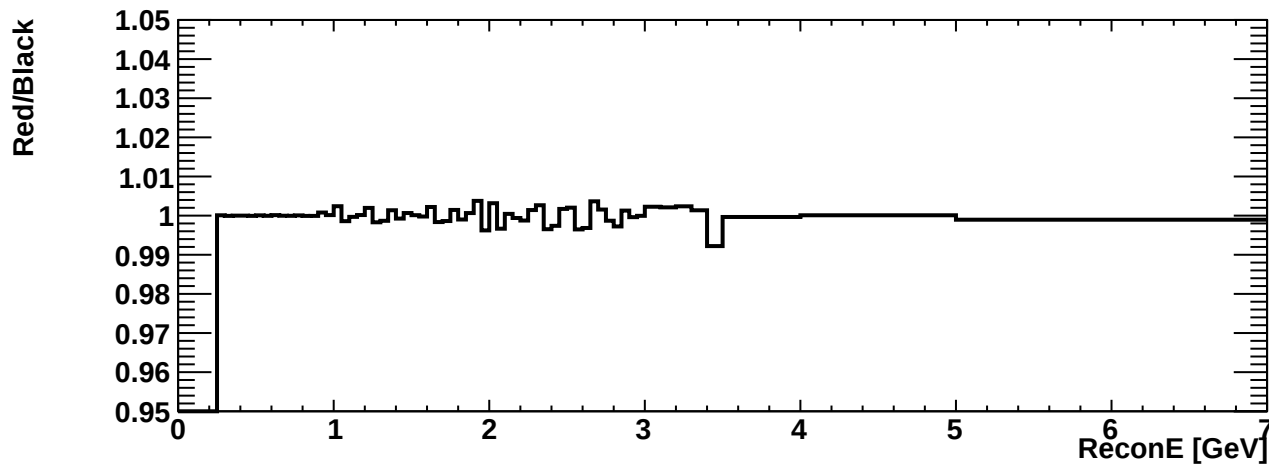
erec_int_numb_ccoth
