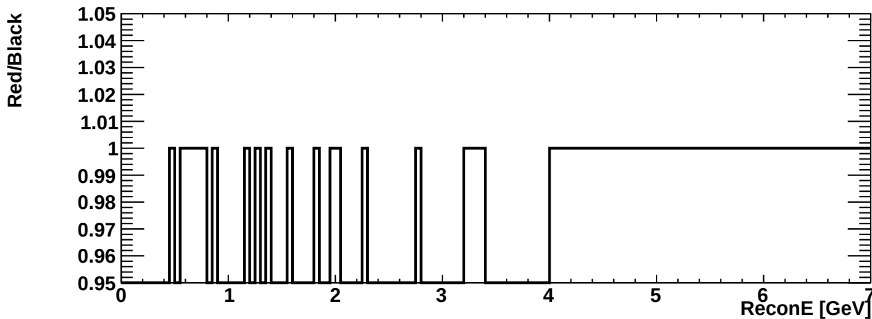
erec_int_nueb_cccoh
