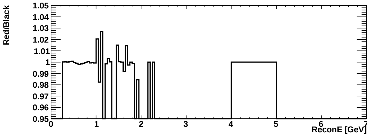
erec_int_nueb_ncpi
