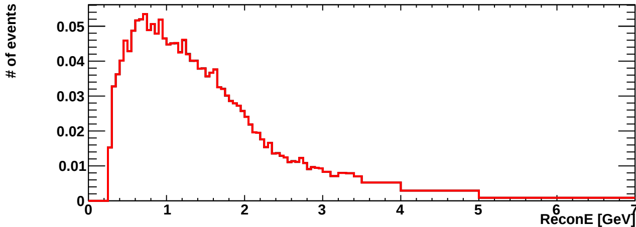
erec_int_numb_ccpi
