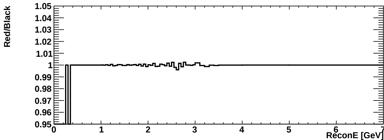
erec_int_nue_ccqe
