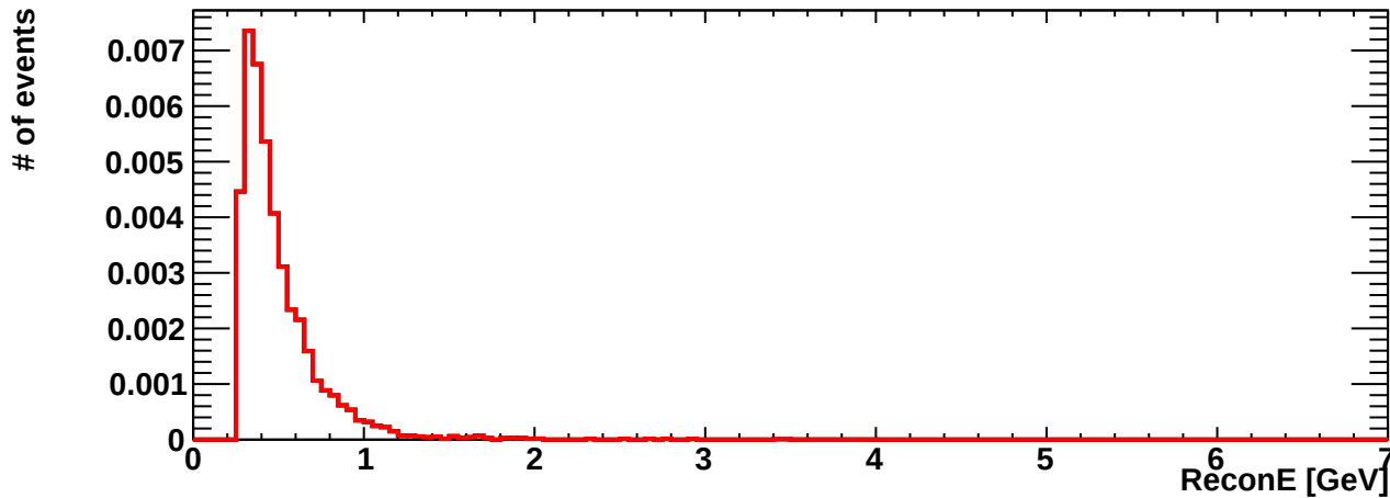
erec_int_nue_ncpi
