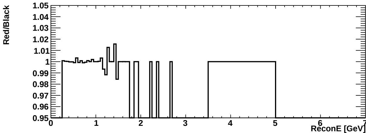
erec_int_numb_ncoth
