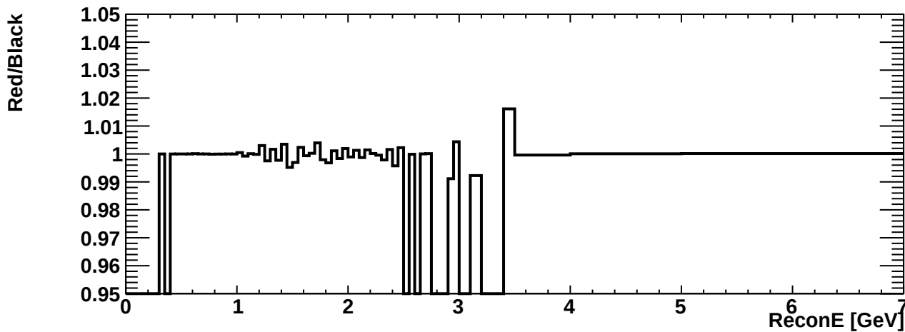
erec_int_nueb_ccqe
