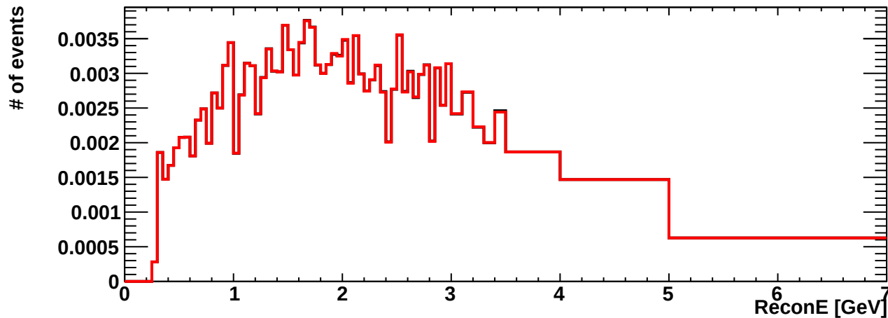
erec_int_numb_ccoth
