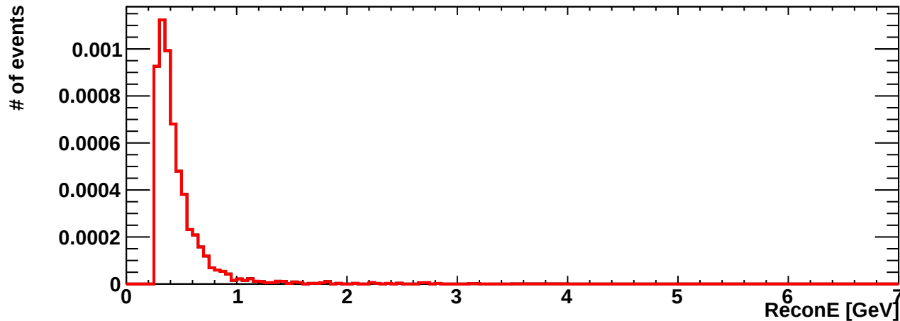
erec_int_nueb_ncoth
