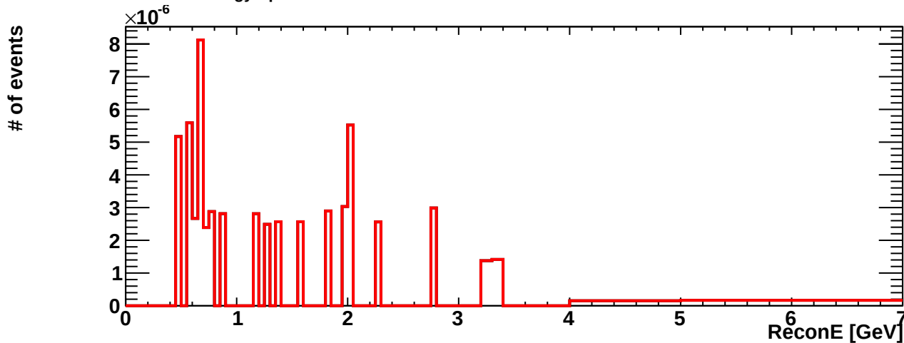
SK nueb ccoch Recon. Energy Spectrum
