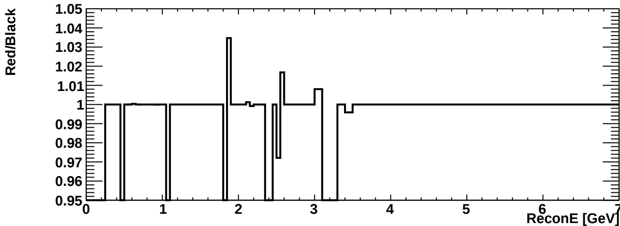
erec_int_nue_ccoth
