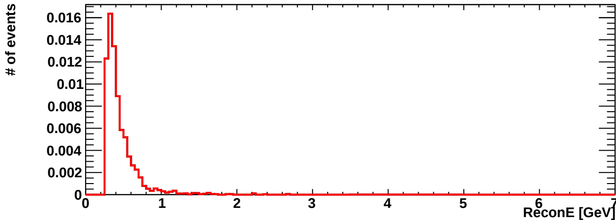
erec_int_numb_ncoth
