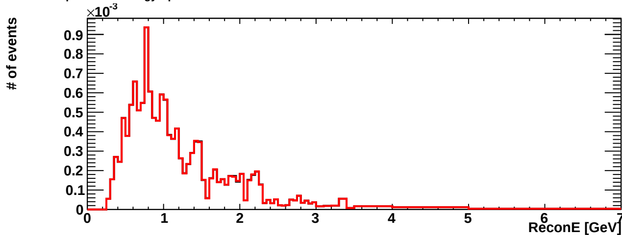
SK nue ccpi Recon. Energy Spectrum
