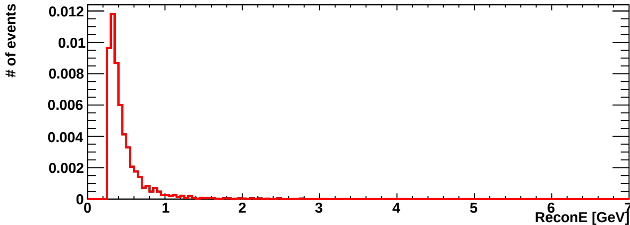
erec_int_nue_ncoth
