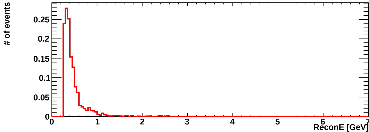
erec_int_numu_ncoth
