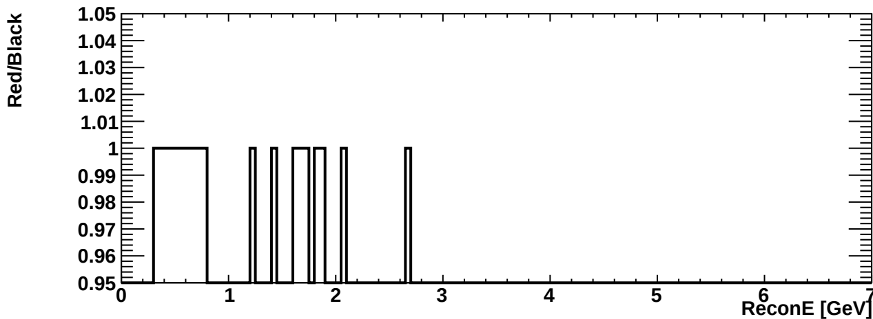
erec_int_nue_cccoh
