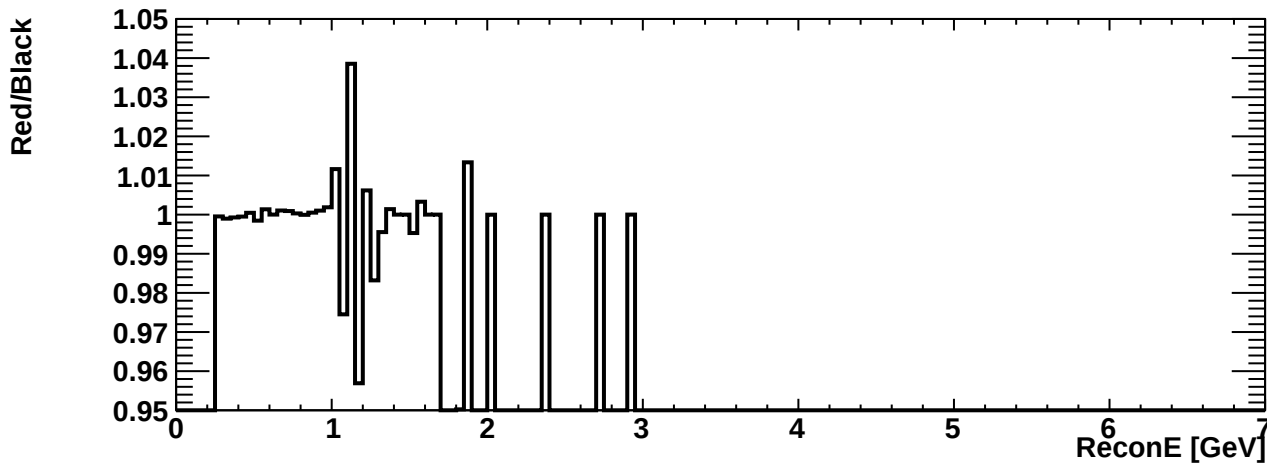
erec_int_numb_ncpi
