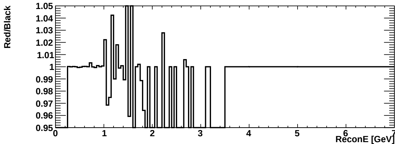
erec_int_nueb_ncoth
