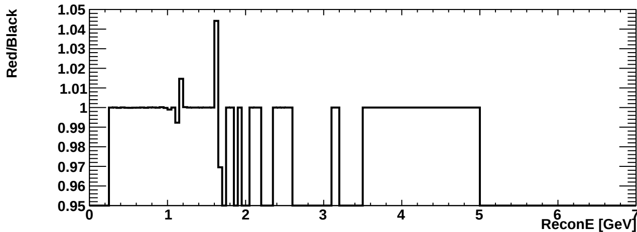
erec_int_numu_ncoth
