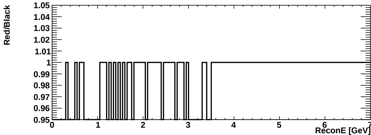
erec_int_nueb_ccoth
