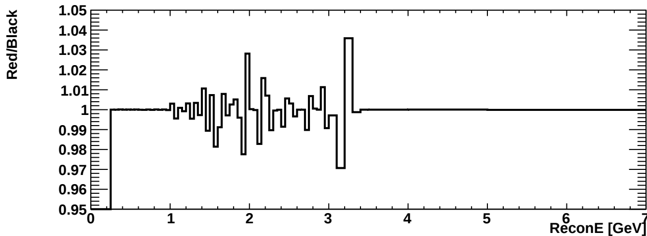
erec_int_nue_ccpi
