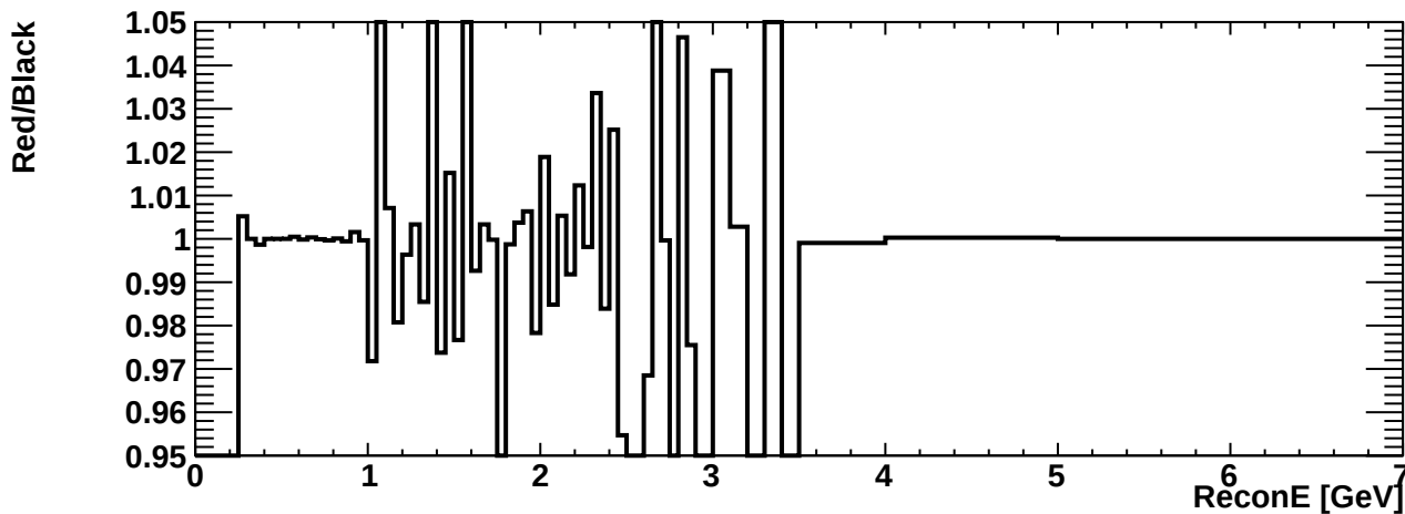
erec_int_nueb_ccpi
