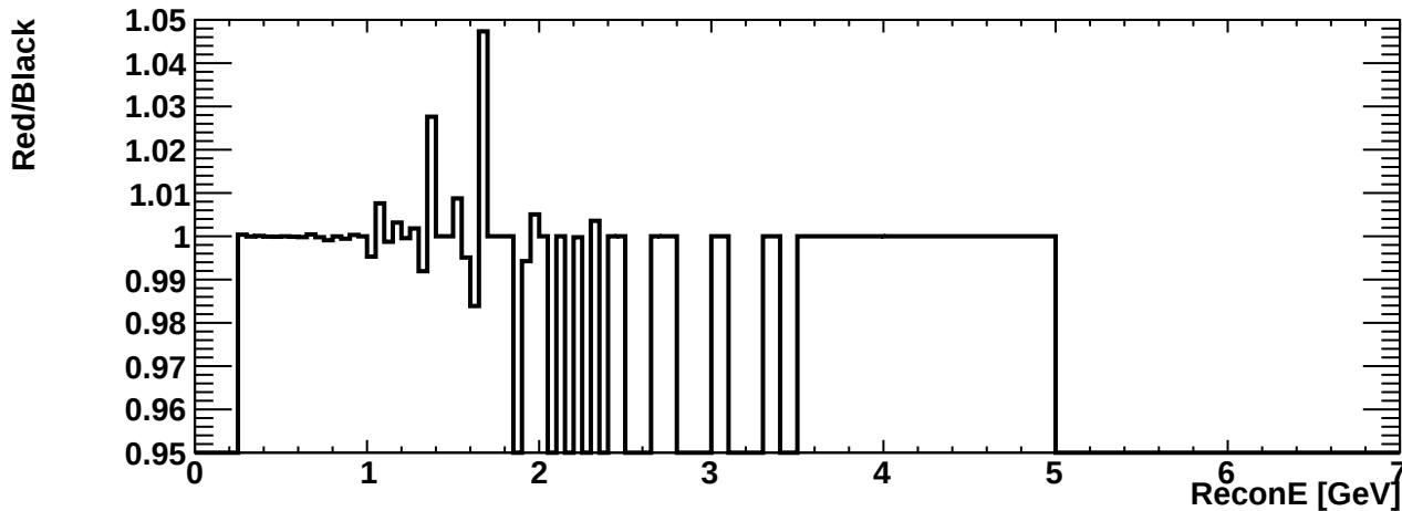
erec_int_nue_ncoth
