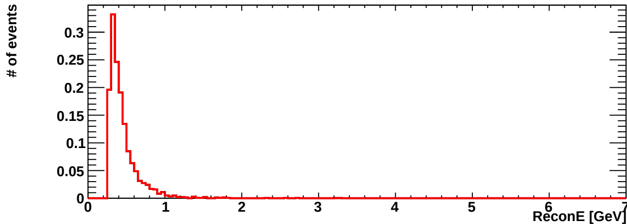
erec_int_numu_ncpi
