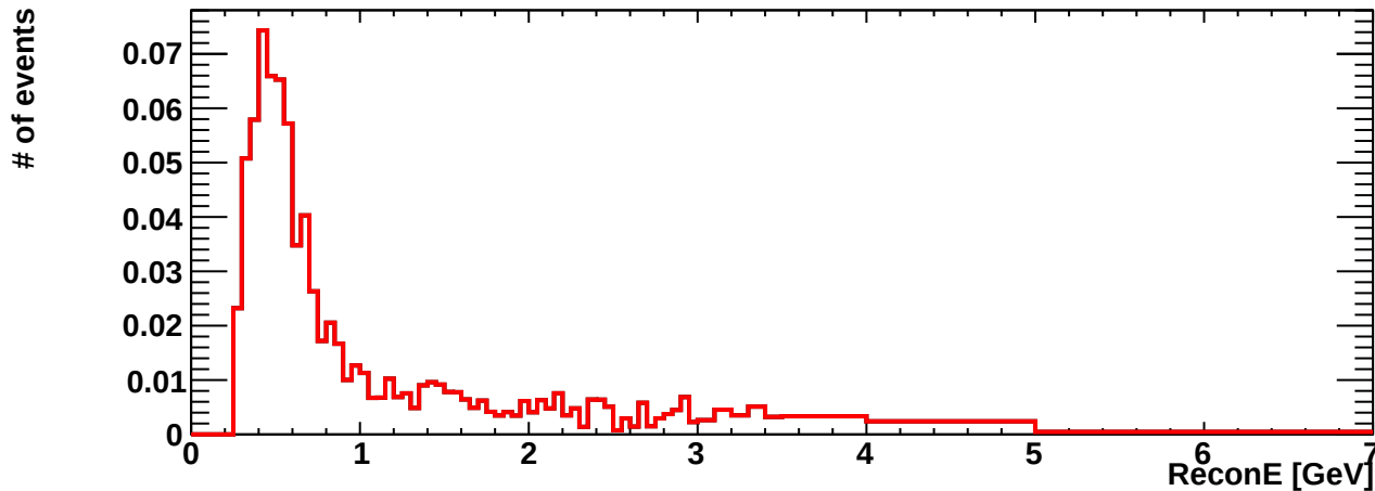
erec_int_numu_cccoh
