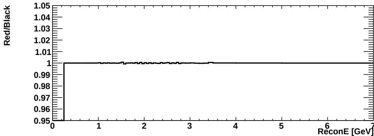
erec_int_numb_ccqe
