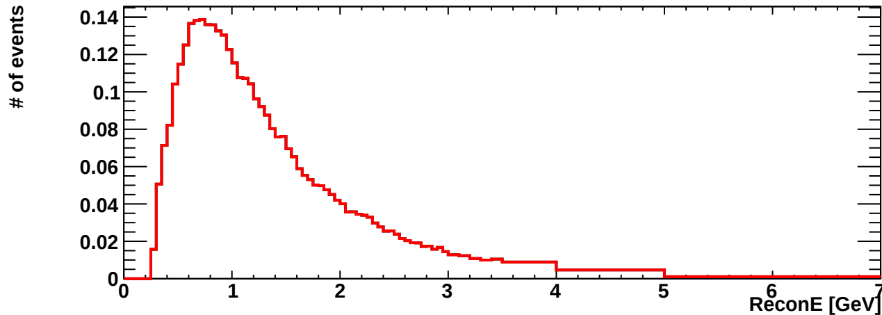
erec_int_numb_ccqe
