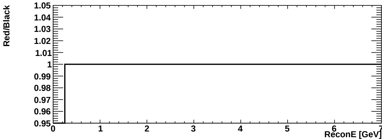
erec_int_numu_cccoh
