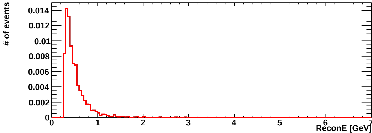
erec_int_numb_ncpi
