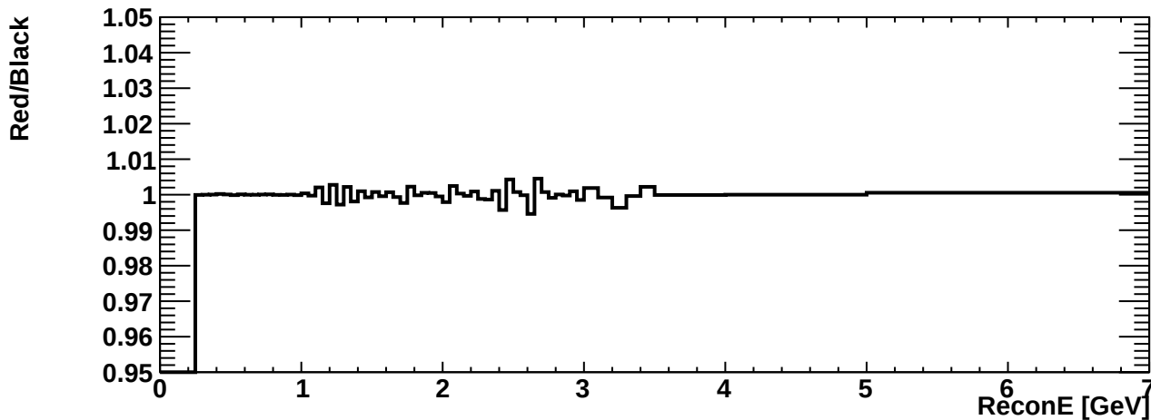
erec_int_numb_ccpi
