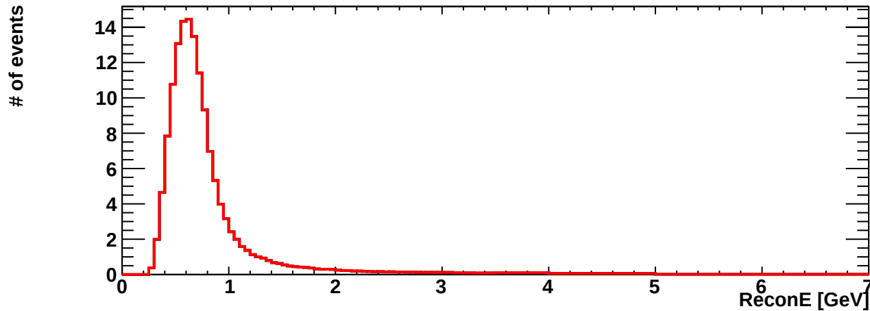
erec_int_numu_ccqe
