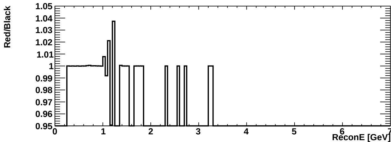
erec_int_numu_ncpi
