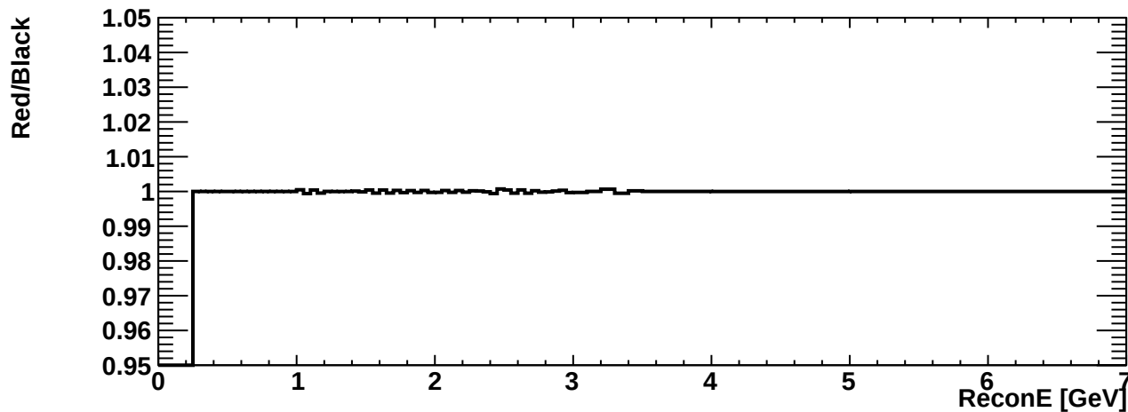
erec_int_numu_ccqe
