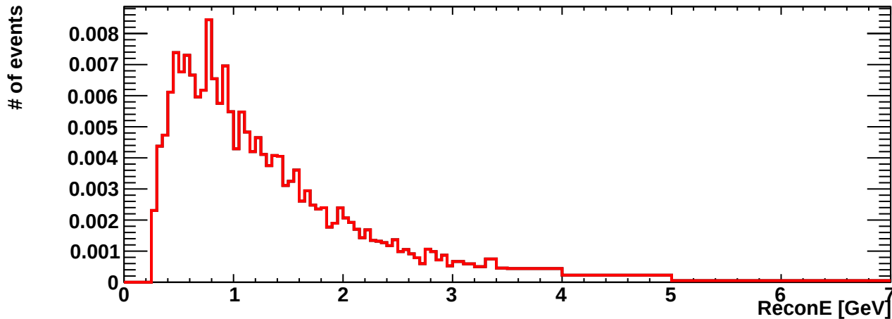
erec_int_numb_cccoh
