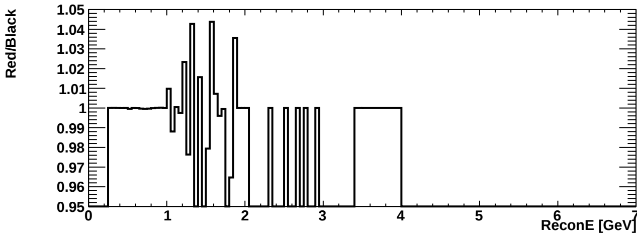
erec_int_nue_ncpi
