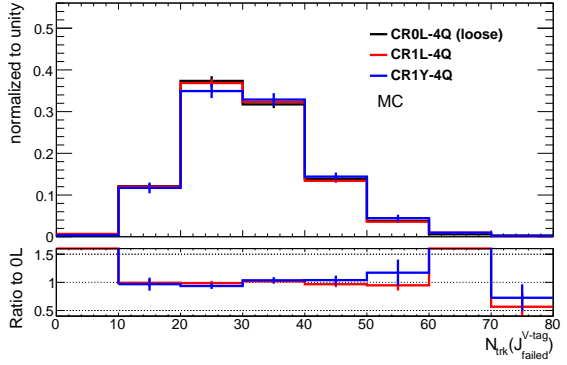
(d) n_{trk}
