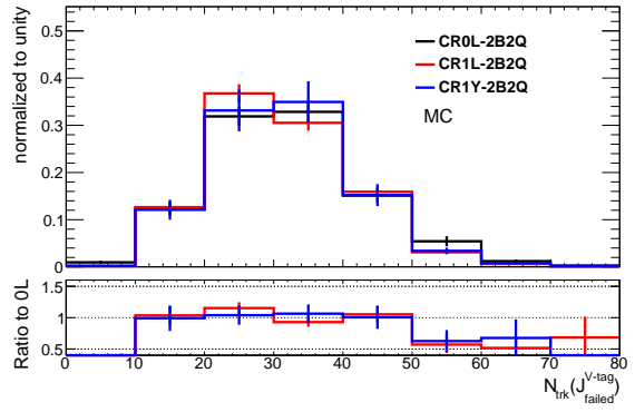
(d) n_{\text{trk}}
