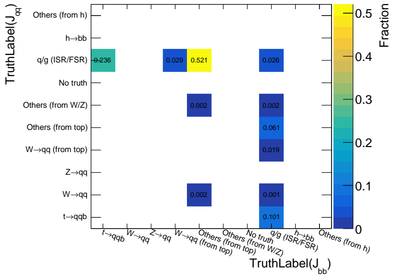
(b) t\bar{t}
