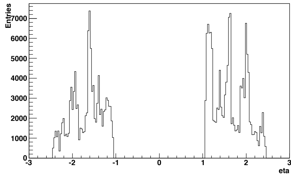
カット後のL1_MU20
