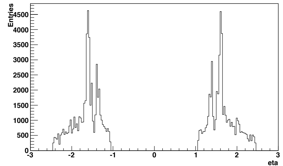
カット後のL1_MU20 (matching のとれた trigger)
