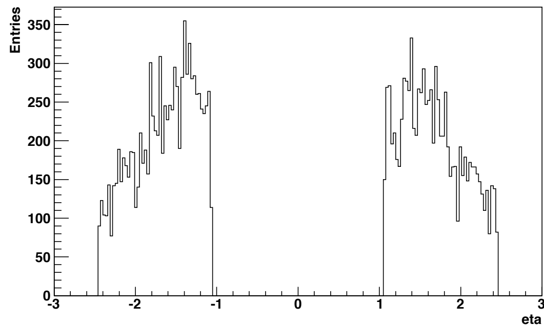
カット後のL1_MU20 (matchingのとれたトリガー (offline p_T > 15 GeV))
