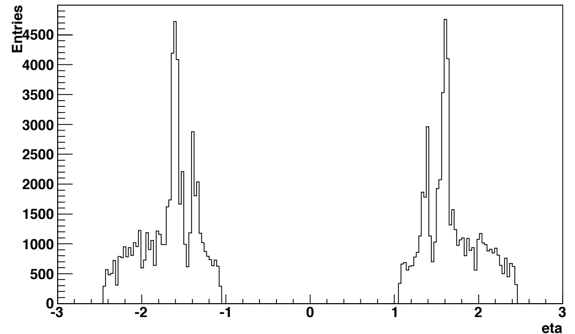
カット後のL1_MU20 (matching のとれた trigger)
