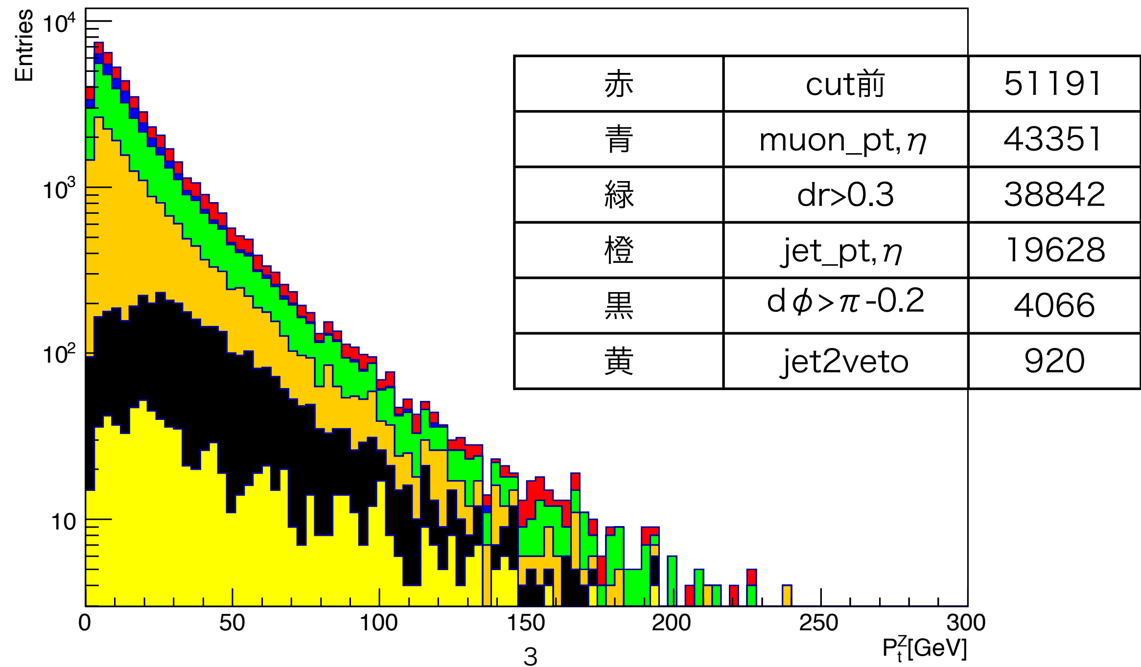
hist_Zpt_noCut
