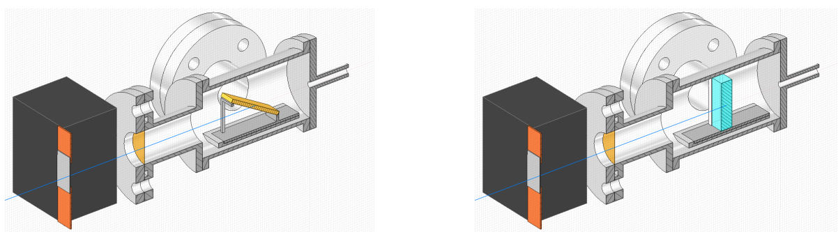
図 2: 真空槽の断面図。左は \text{SiO}_2 粉末標的を使う場合、右は \text{SiO}_2 エアロジェル標的を使う場合。真空槽の直前にあるのは Al ディグレーダ (灰色) と Cu コリメータ (銅色)、鉛ブロック (黒色)。
