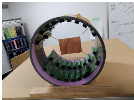
図 3: 昨年度使用した磁石。中央の銅板の位置に垂直方向に約 60 G の一様磁場を発生させる。
