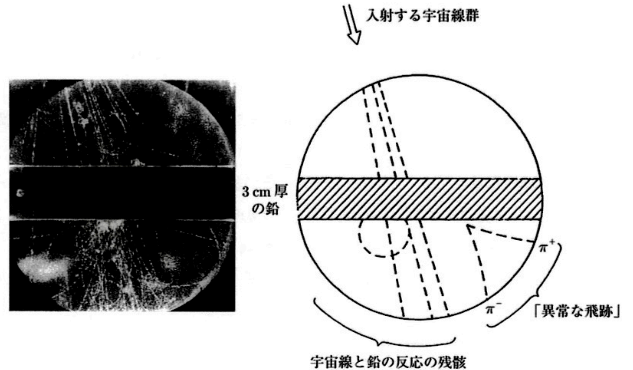
図 1.7 最初のストレンジ粒子. 宇宙線が鉛の板に当たり, K^0 が生成され, その K^0 は荷電パイ中間子対に崩壊している (写真著作権: Prof. Rochester, G. D.: Nature, 160, 855 (1947). 版權: Macmillan Journals)
